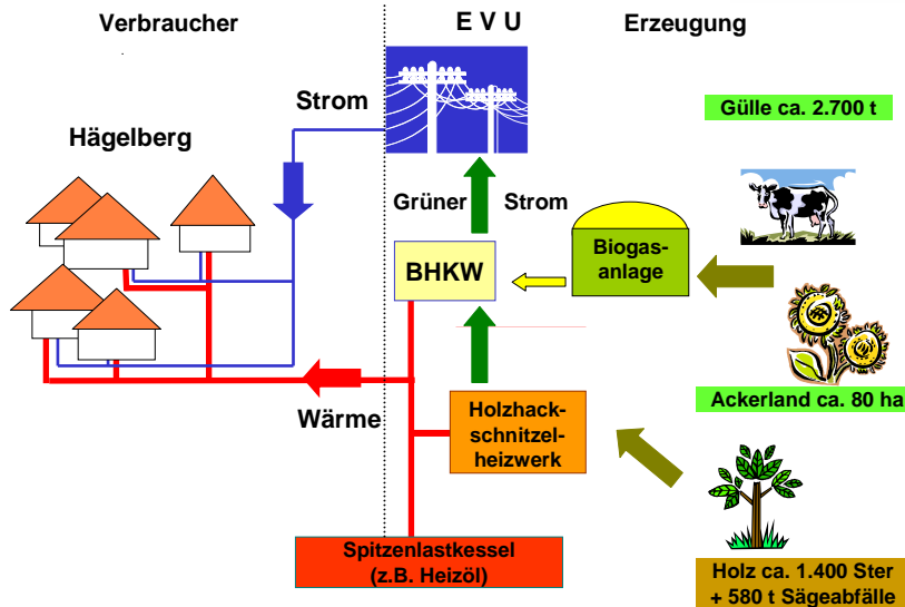
Anlagenschema für Nahwärmever-sorgung Hägelberg
