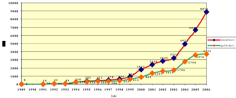
Installierte & geförderte Leistung Fotovoltaik seit 1989 in Freiburg (kWp) Stand Dezember 2006
